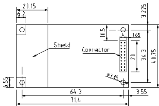
TOP VIEW (Unit:mm)
